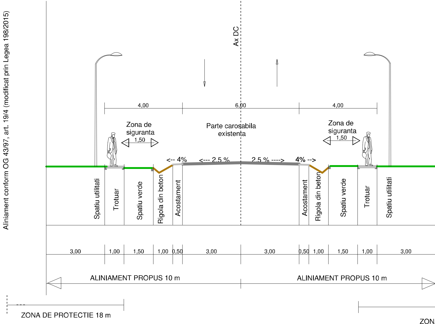
PROFIL TRANSVERSAL PROPUȘ PENTRU DC IN INTRAVILAN SCARA 1:100
