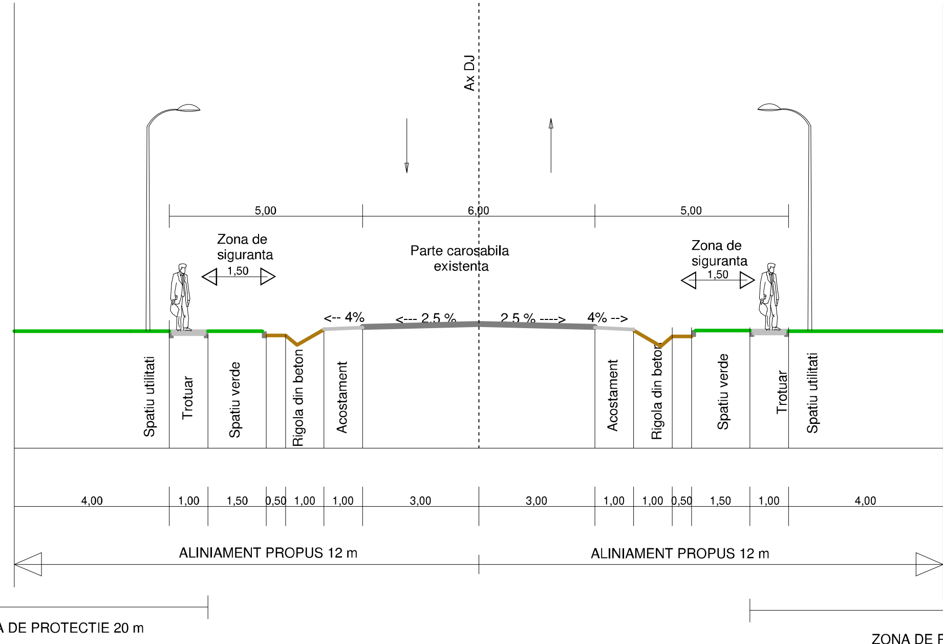
PROFIL TRANSVERSAL PROPUȘ PENTRU DJ IN INTRAVILAN SCARA 1:100
